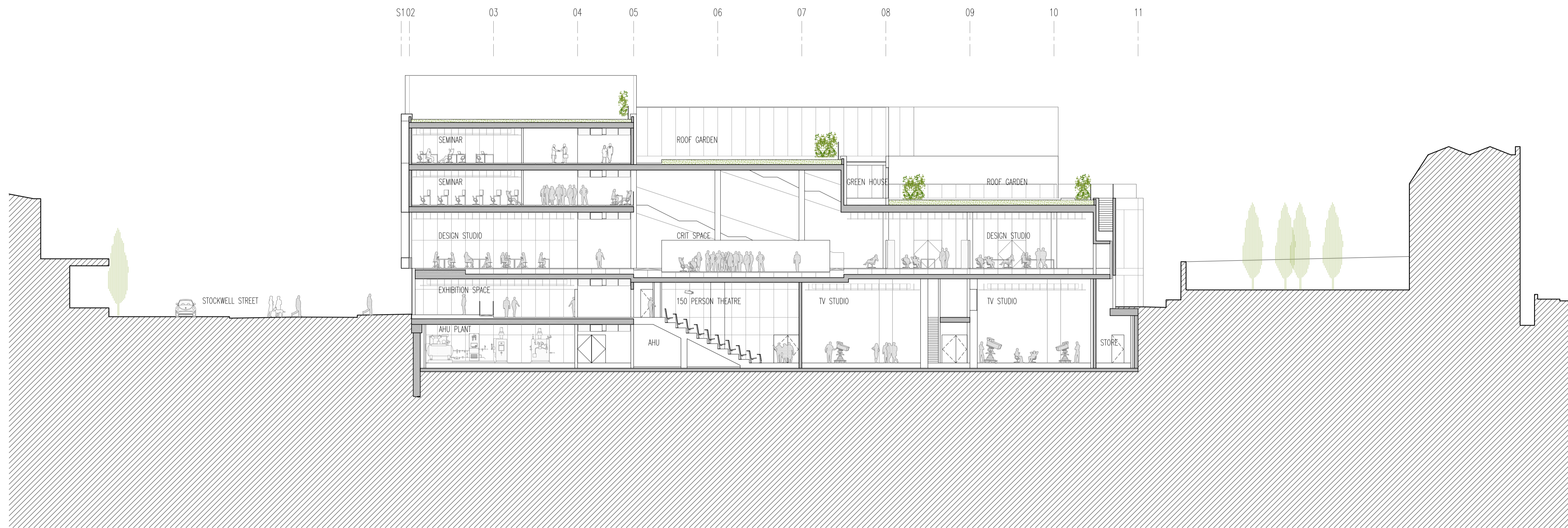
02 LONG SECTION B-B 1:200
