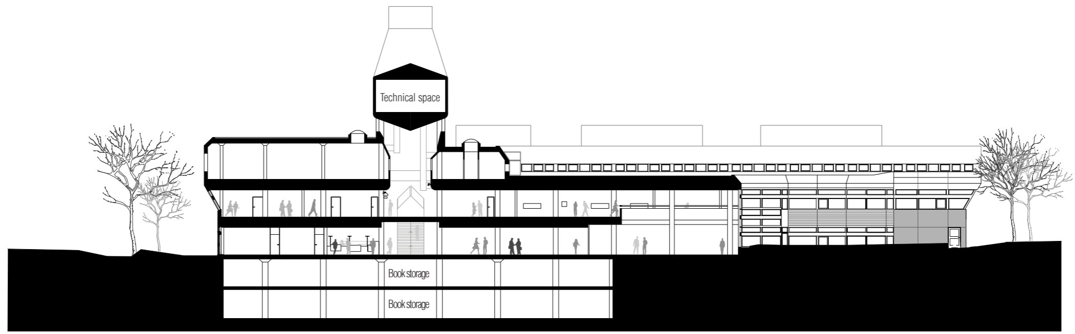
Section BB 1:400
